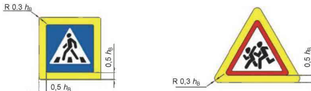
Рисунок 12 — Приклад знаків із додатковою світлоповертальною зовнішньою облямівкою жовтого кольору
