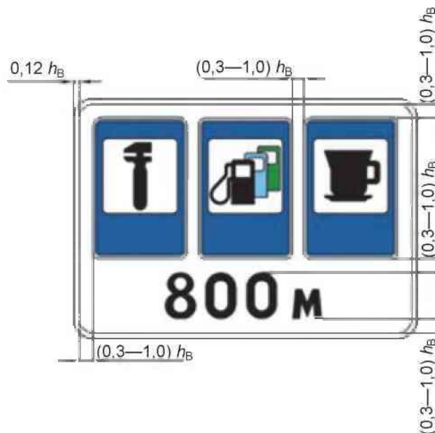
Рисунк 10 — Приклад розміщення знаків на щиті прямокутної форми з білим світлоповертальним тлом
